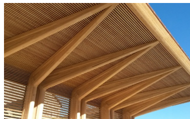
Vue détaillée de la toiture
