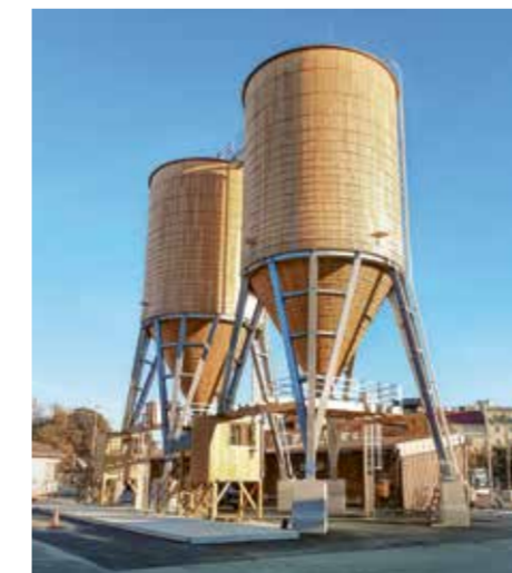
Deux silos en bois rond d'une capacité de 500 m 3 chacun dans la ville de Vienne.
